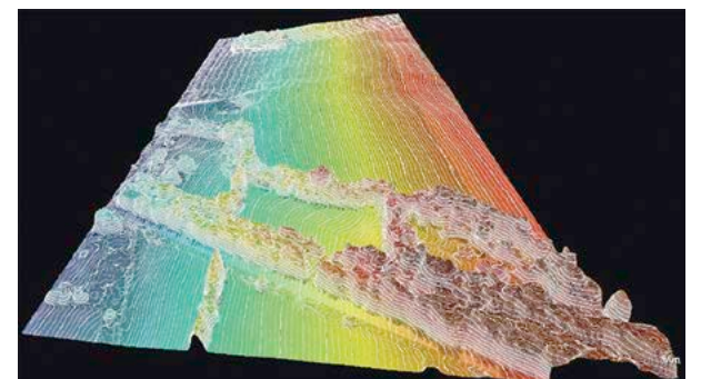
Figure 3 - Carte de courbes de niveau superposée au modèle 3D, illustrant le relief par des lignes reliant des points d'altitude égale. Elle indique les hauteurs du sol par rapport au niveau moyen de la mer et permet de repérer les cuvettes, d'anticiper l'érosion liée au ruissellement et de mieux gérer les milieux humides.
